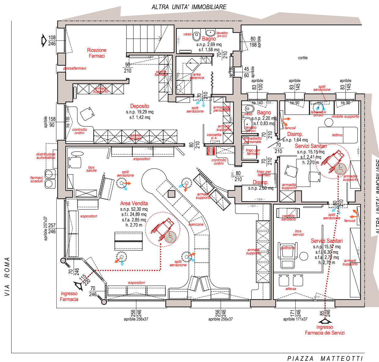
PIANTA PIANO TERRA · 1:100
